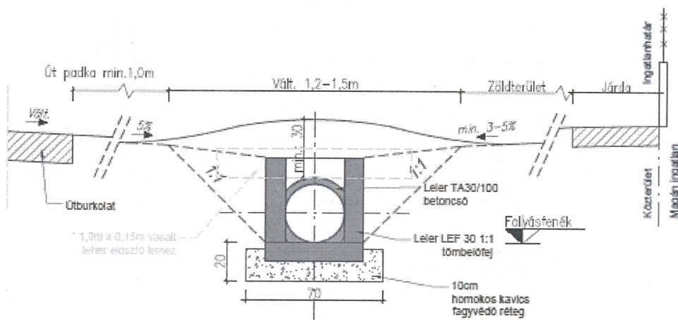
A-A metszet
